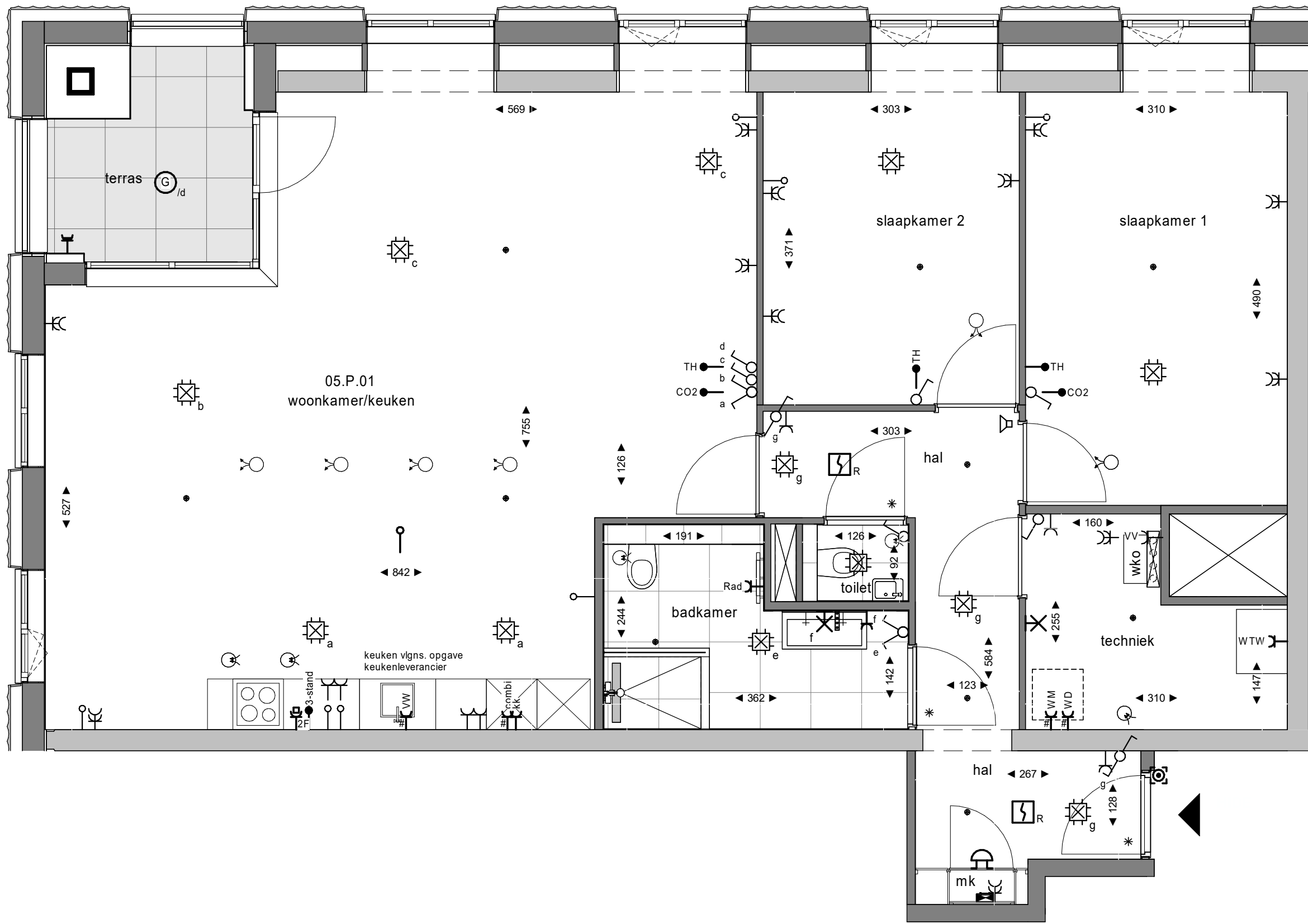
plattegrond 1 : 50 5e verdieping
