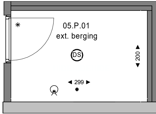
plattegrond berging 1 : 50 5e verdieping
